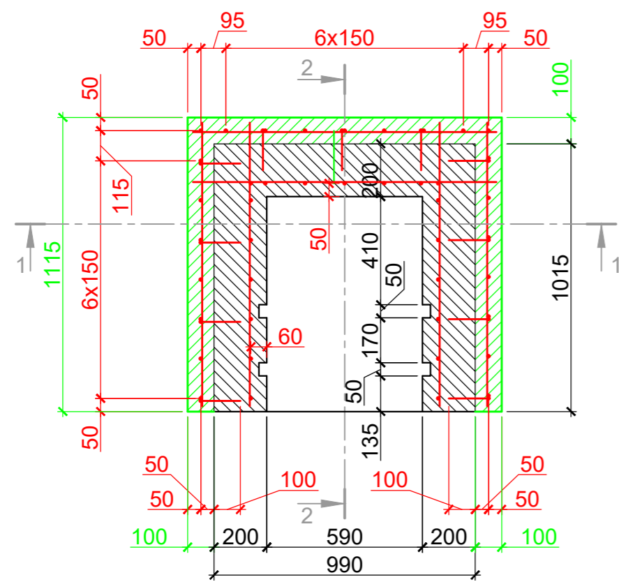
Griezums3-3 M 1:20
