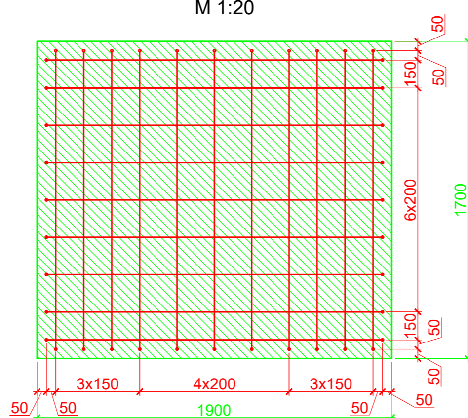
Apakšējā stiebrojuma shēma M 1:20
