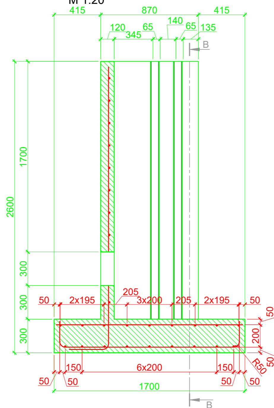
Griezums A-A M 1:20
