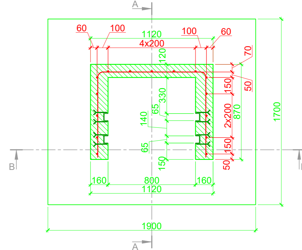
Plāns M 1:20
