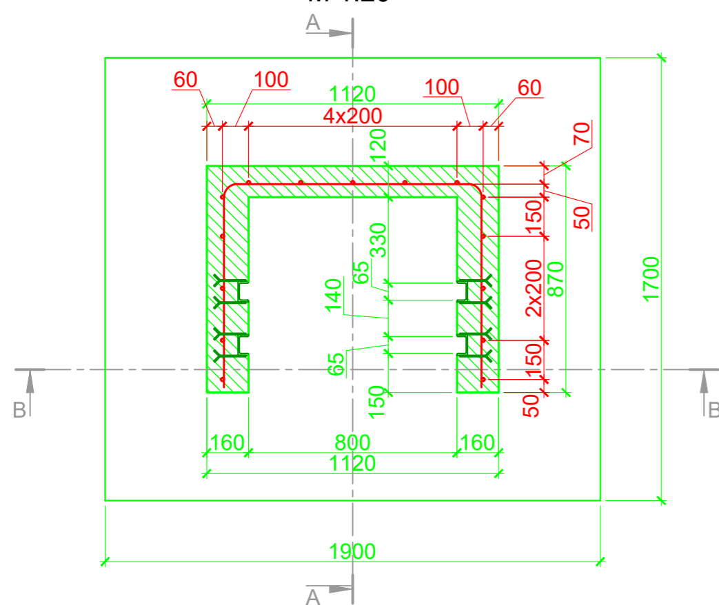
Plāns M 1:20
